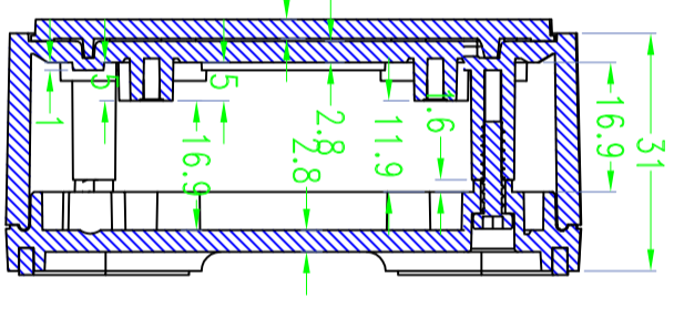
SEC D-D
